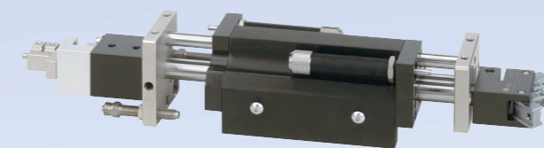
GZ 20 / VE 25 Greifzange mit Vertikal-Element Pince avec élément linéaire Mano di presa con unità lineare Gripper with linear element
