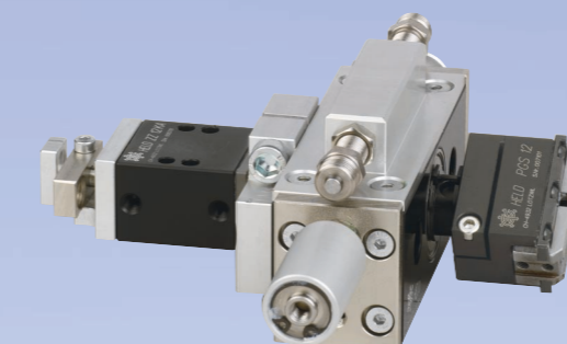
PGS 12 KA / DA 12 2M Parallel-Greifzange drehbar Pince parallèle rotative Mano di presa parallela rotante Parallel gripper rotary
